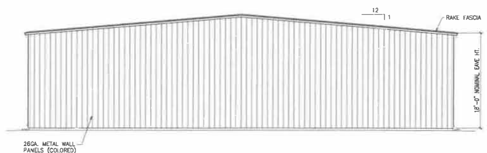
WEST/REAR ELEVATION SCALE: 1/8"=1'-0"
