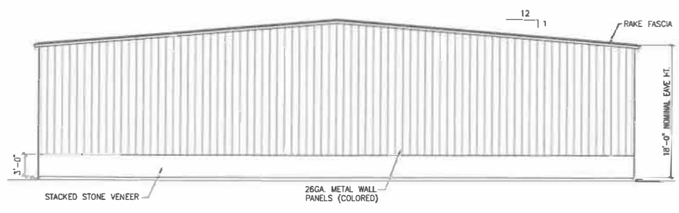
EAST/FRONT ELEVATION SCALE: 1/8"=1'-0"
